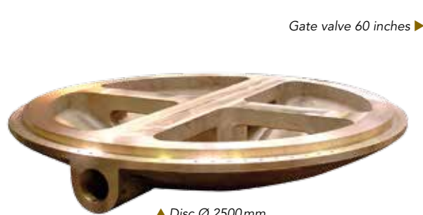
▲ Disc Ø 2500mm
